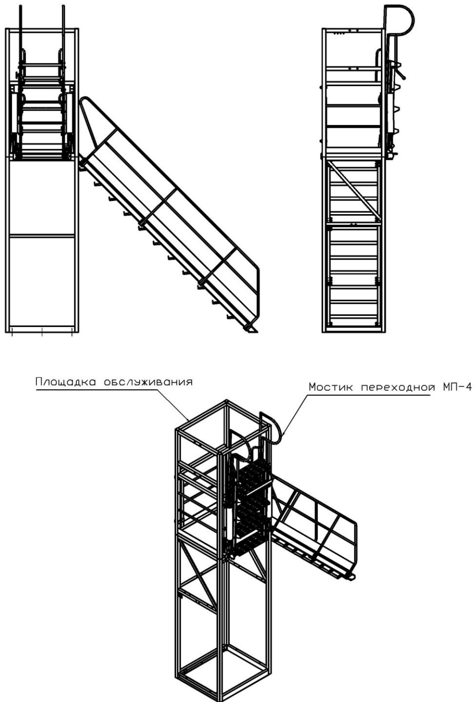
Рисунок 2 - Площадка обслуживания с переходным мостиком
