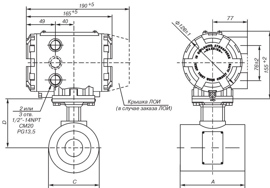
Рис.7. Расходомер Rosemount 8700 с датчиком расхода 8711 (Диу от 40 до 200) и преобразователем 8732E (размеры см.табл.11).
