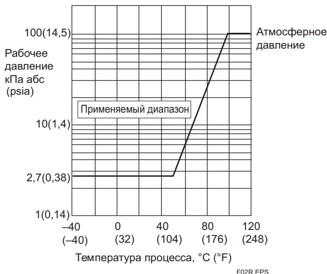
Рис. 1-2. Температура процесса и рабочее давление [для модели EJA530E]
